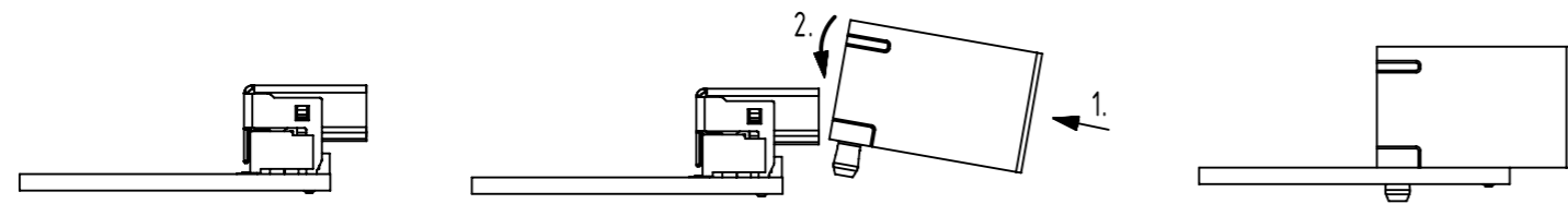
soldered Mini DisplayPort receptacle
