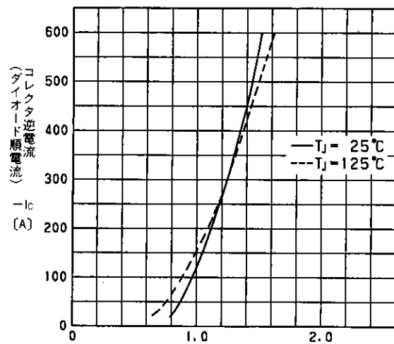
エミッタ・コレクタ間電圧 V_{cco} (V) (ダイオード順電圧) 高速フリーホイーリングダイオード順電圧特性 Forward Voltage of Free Wheeling Diode
