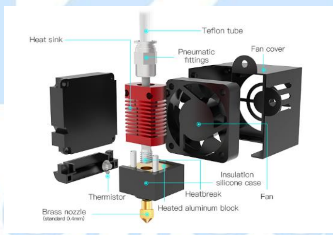
Vista explosionada
