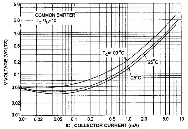
V_{ce(sat)} - I_c
