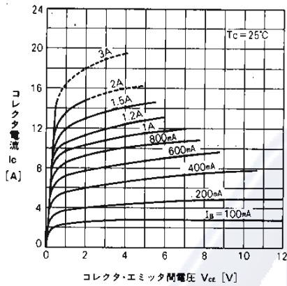
出力特性
