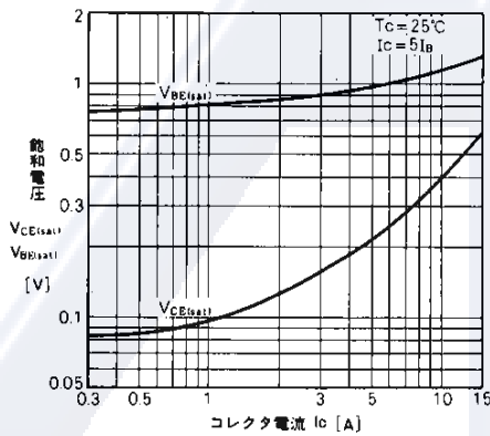
飽和電圧—コレクタ電流特性
