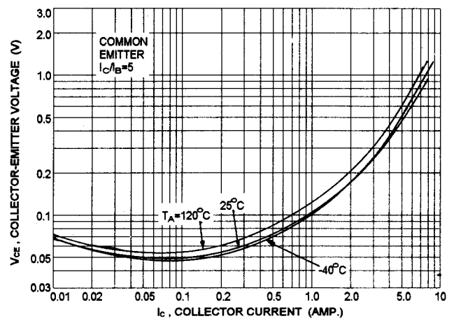
V_{CE} - I_C
