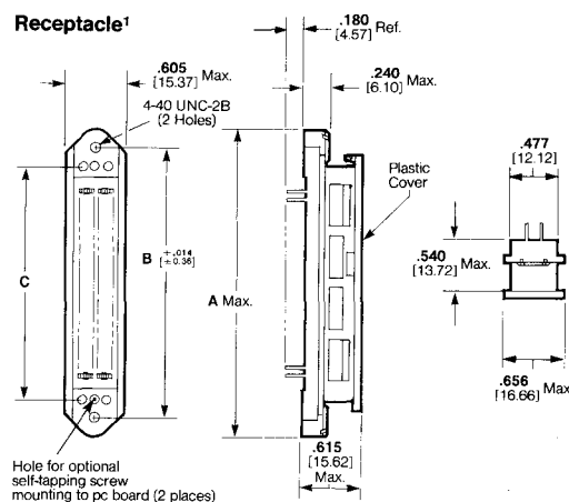
Receptacle 1
