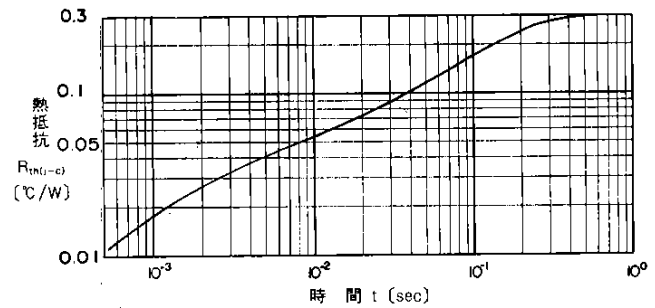
過渡熱抵抗(トランジスタ)特性
