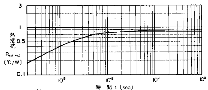
過渡熱抵抗(ダイオード)特性
