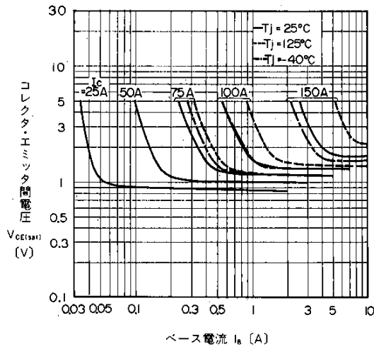
出力特性
