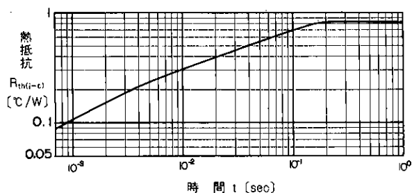
過渡熱抵抗(トランジスタ)特性
