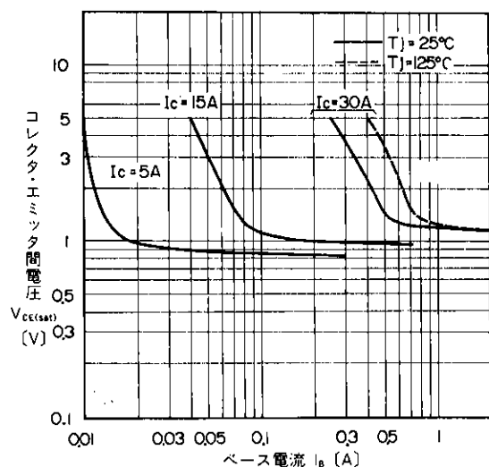
出力特性
