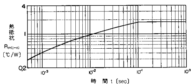
過渡熱抵抗(ダイオード)特性
