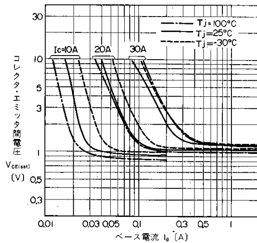
出力特性
