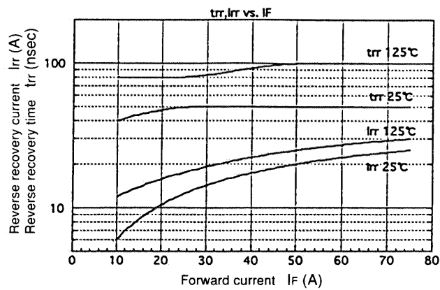
逆回復時間、逆回復電流—逆回復特性 Reverse recovery characteristics t_{rr} , I_{rr} vs. I_F
