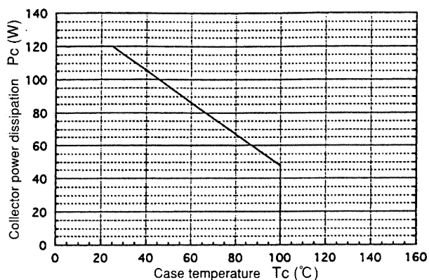
IGBT 電力低減特性 Power derating for IGBT(per device)
