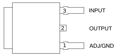
TO252-2 (5)
