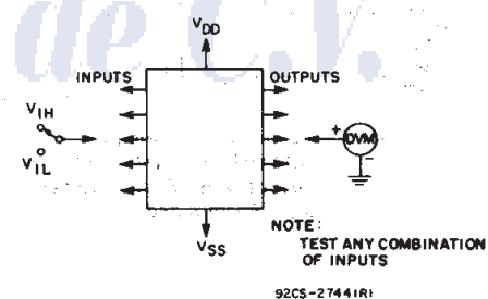
Fig. 25—Input-voltage test circuit.
