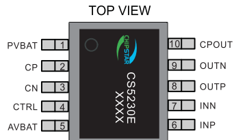
CS5230E(ESOP10 PACKAGE)
