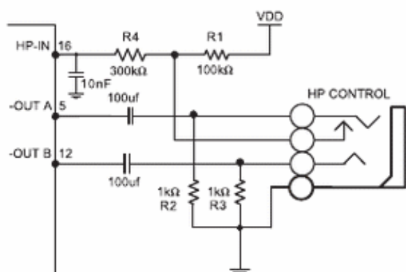
立体耳机工作电路示意图
