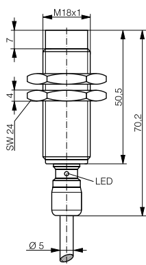
DW-LD-71x-M18
