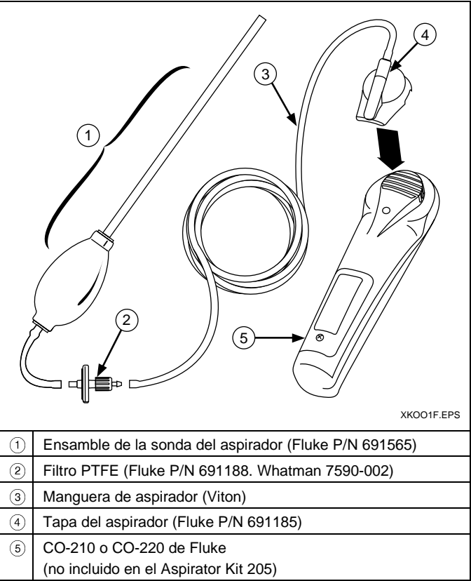
Figura 1. Aspirator Kit (Juego de aspirador) CO-205
