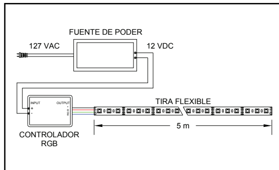
Diagrama básico de conexión
