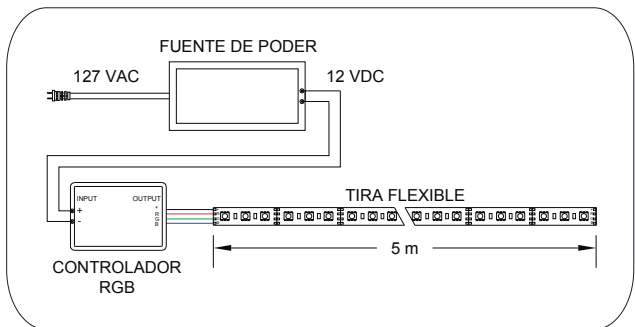
Diagrama de conexión básica
