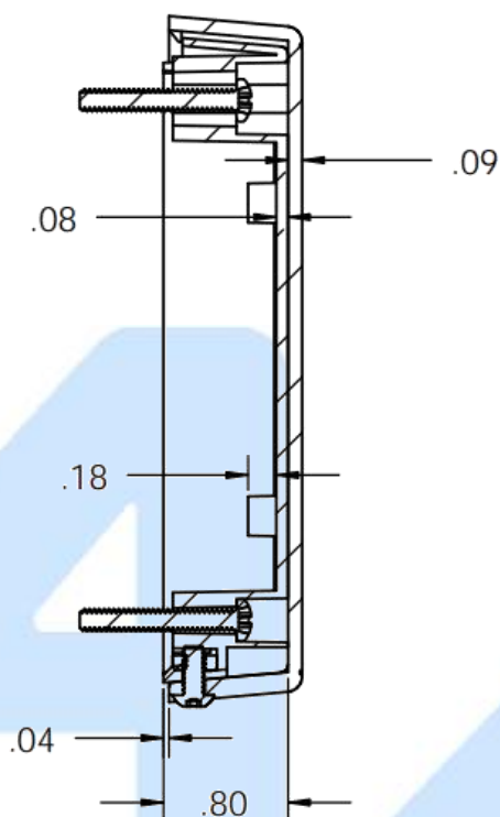
Vista seccionada de la bandeja de montaje
