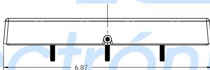
Vista lateral de la bandeja de montaje
