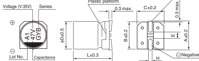
(φ6.3) 【Standard】
