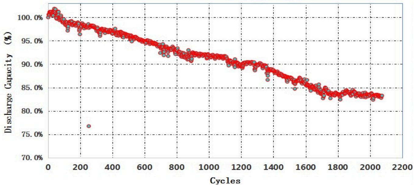
HDCF26650-3400mAh-3.2V (3C) 循环曲线图
