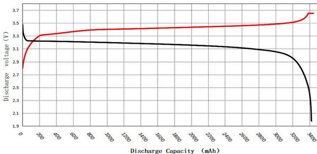
HDCF26650-3400mAh-3.2V (3C) 充放电曲线
