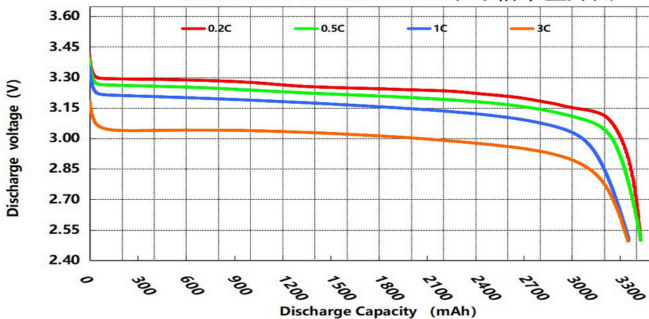
HDCF26650-3400mAh-3.2V (3C) 倍率温升图
