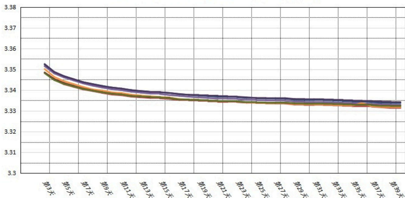
HDCF26650-3400mAh-3.2V (3C) 自放电
