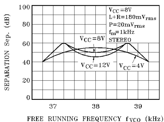
Sep. - f_{VCO}
