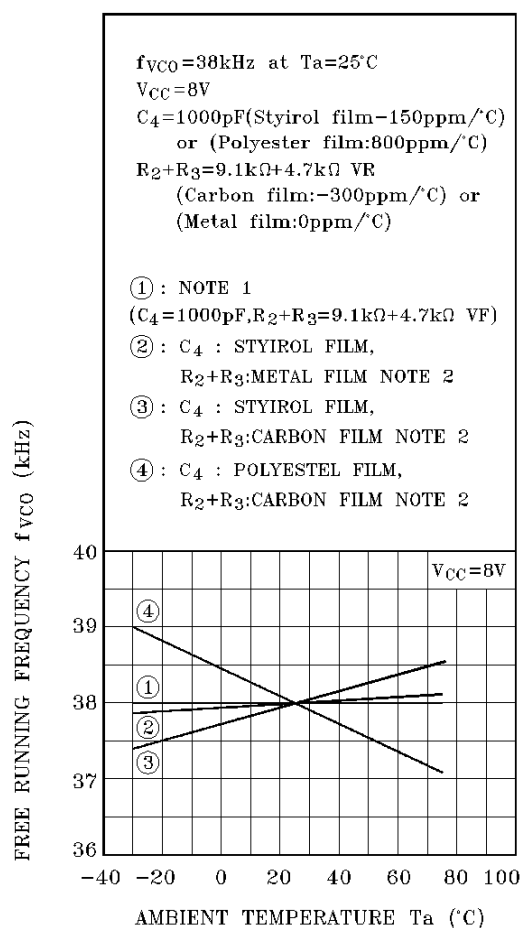
f_{VCO} - T_a
