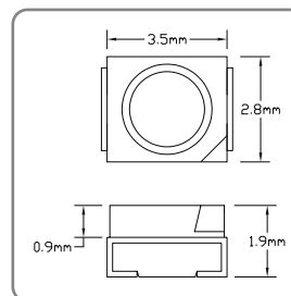
Dimensiones
