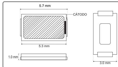
Dimensiones
