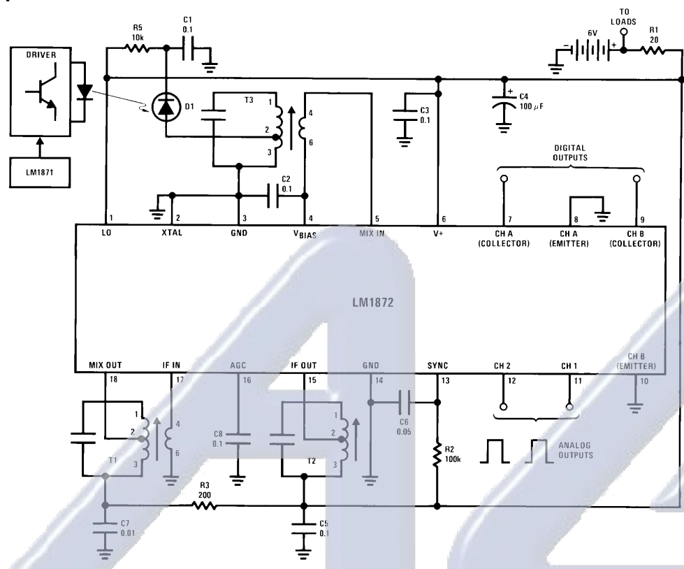
Bottom View FIGURE 9a. IR Type Data Link
