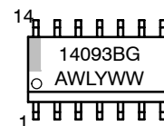
SOIC-14 D SUFFIX CASE 751A
