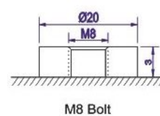
M8 Bolt
