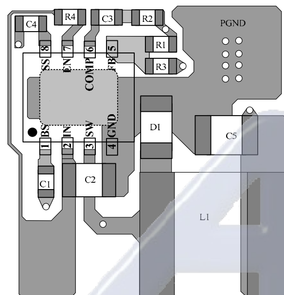
TOP Layer
