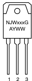
TO-3P CASE 340AB STYLES 1,2,3
