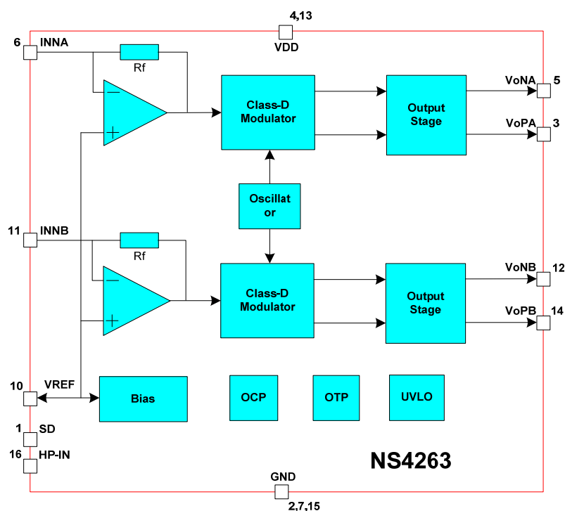
图4 NS4263 原理框图(上图标号为 SOP16 封装)
