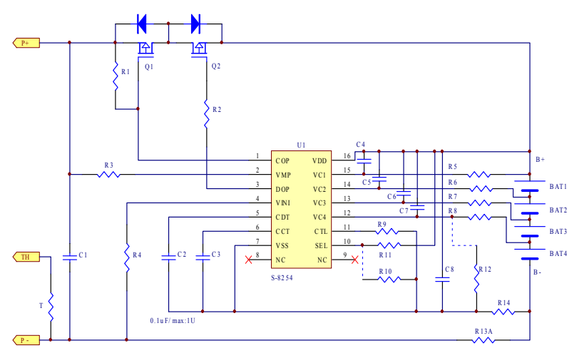
Schematic diagram 原理图：
