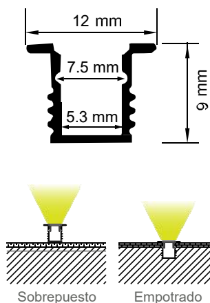
PERFIL-ACCESORIOS-870
