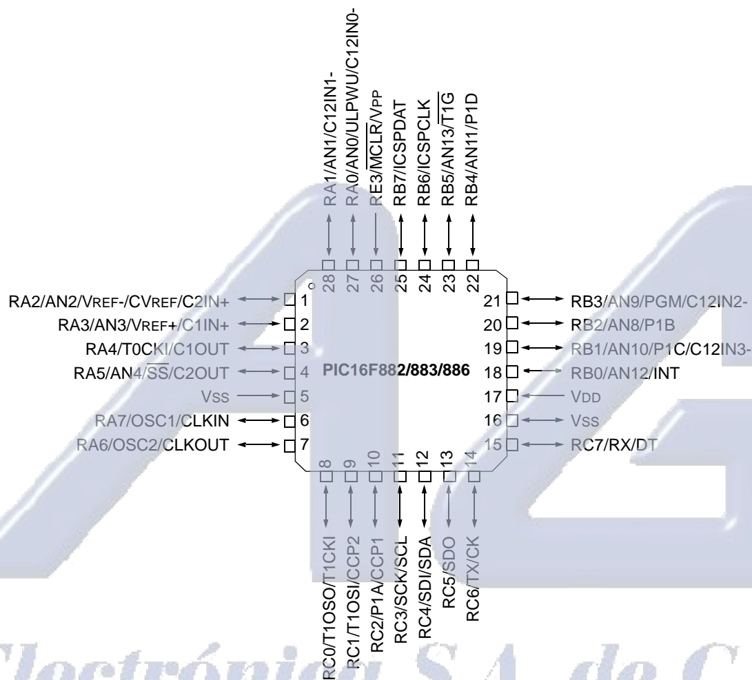
28-pin QFN
