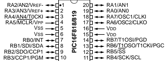
20-Pin SSOP
