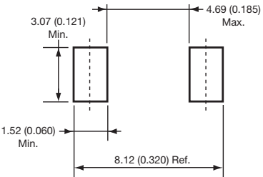
DO-214AB (SMC)
