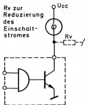
Lampentreiber
