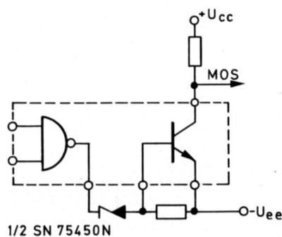
300 mA-Leistungsschalter mit variablem Bezugspotential
