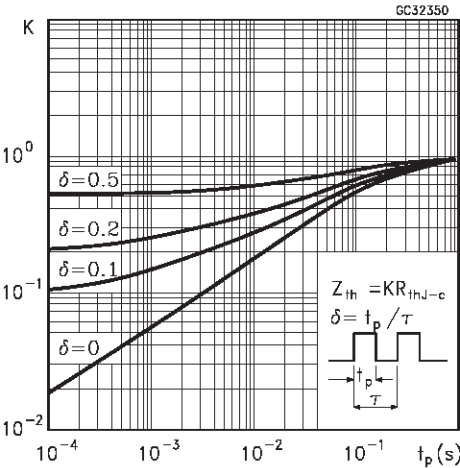
Thermal Impedance
