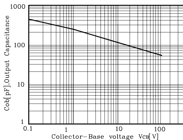
Fig. 6 C_{ob} - V_{CB}
