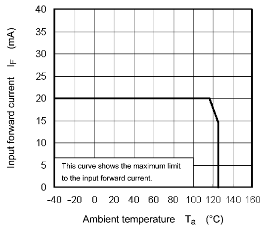
Fig. 13.2.2 I_F - T_a
