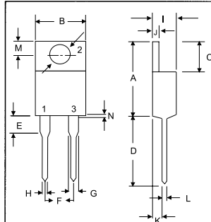
TO-220A
