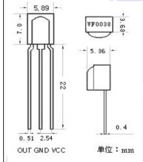
外型尺寸及引脚排列图
