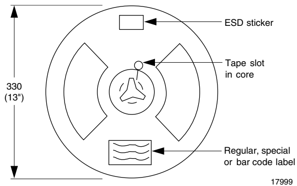
Fig. 22 - Reel Dimensions
