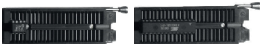
(a) Inserción de un 93LC46
